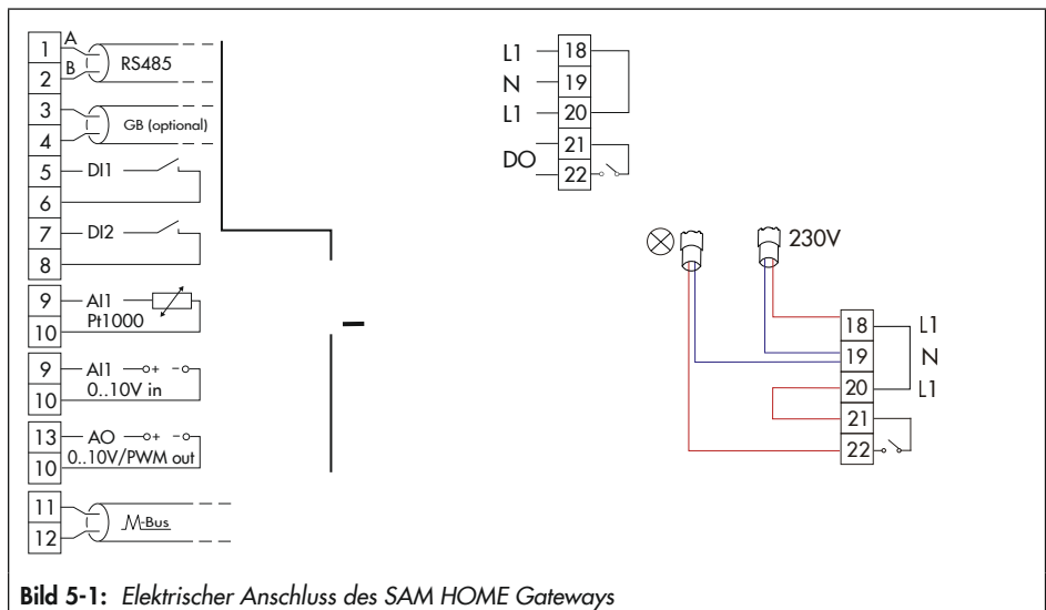
Bild 5-1: Elektrischer Anschluss des SAM HOME Gateways
