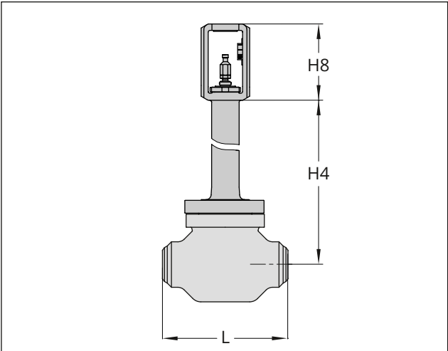
Fig. 8: Tipo 3251/3251-AM soffietto o parte isolante
