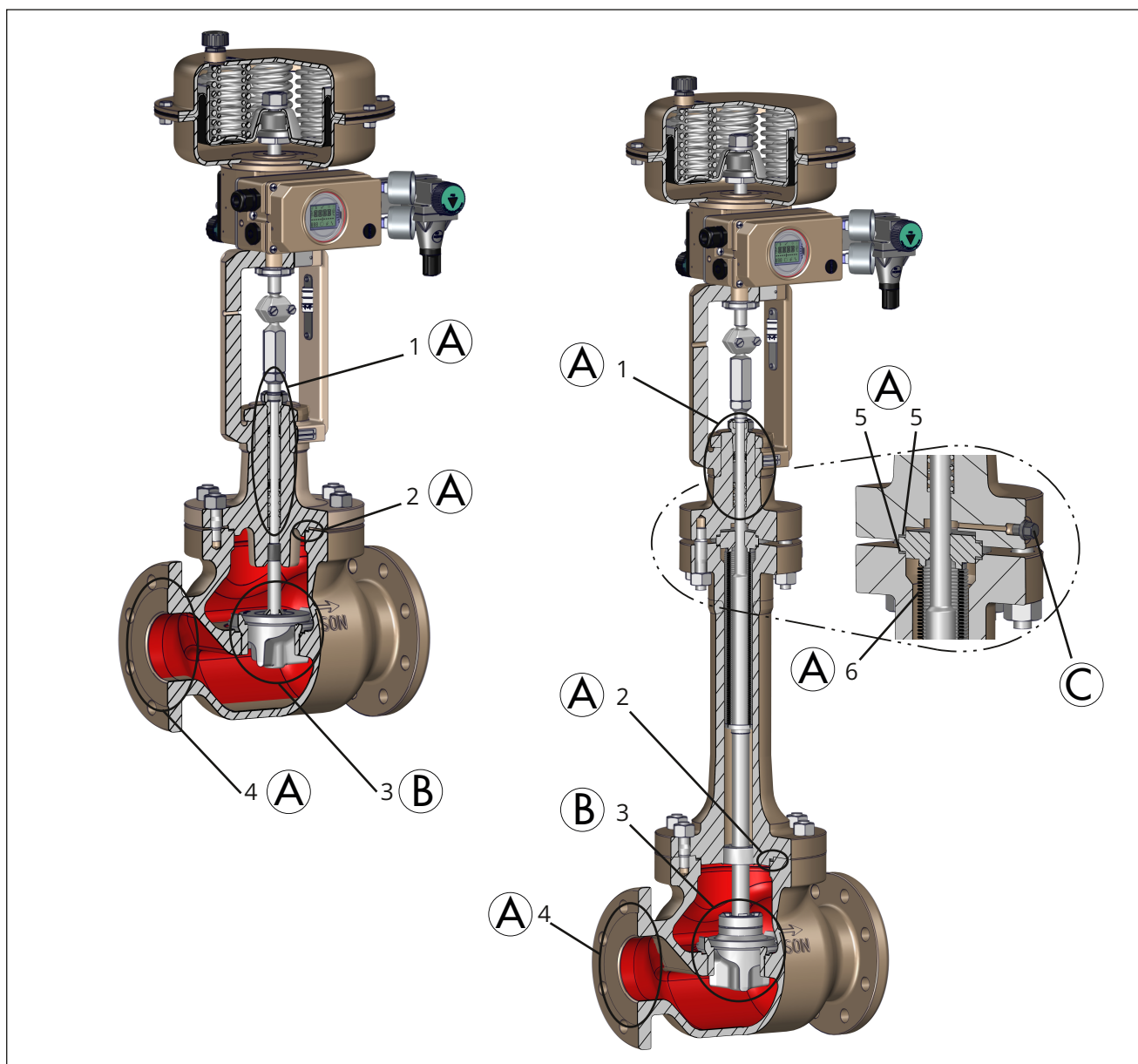
Fig. 22: Possibili punti di perdita nella valvola di controllo (esempi: a sinistra versione con parte superiore standard, a destra versione con soffietto, rappresentativa anche delle versioni con parte isolante o adattatore).
