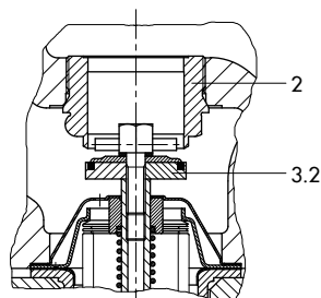
Obturador con junta blanda
