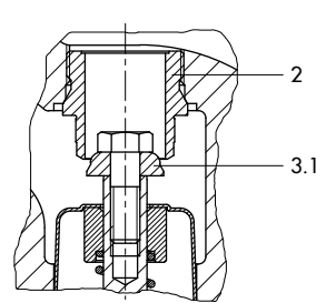
Obturador para peque- ños caudales, K_{VS} \leq 2,5 sin fuelle de compensación
