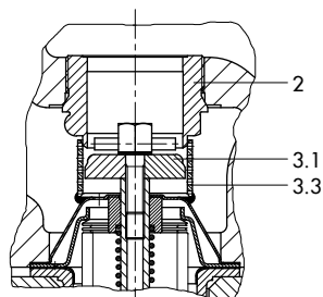
Obturador de cie- rra metálico, con di- visor de flujo ST1
