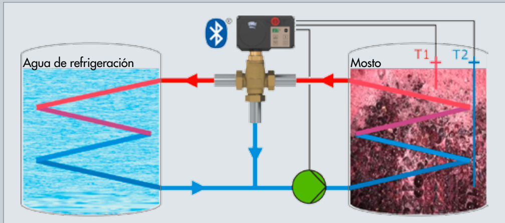
Regulación con punto de consigna fijo con medición de la media, control de bomba y ajuste del punto de consigna en el equipo
